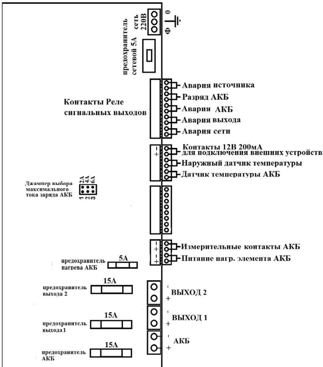
Рисунок 4. Органы управления и коммутации.
