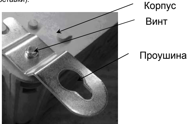
Рисунок 3. крепление проушин.
